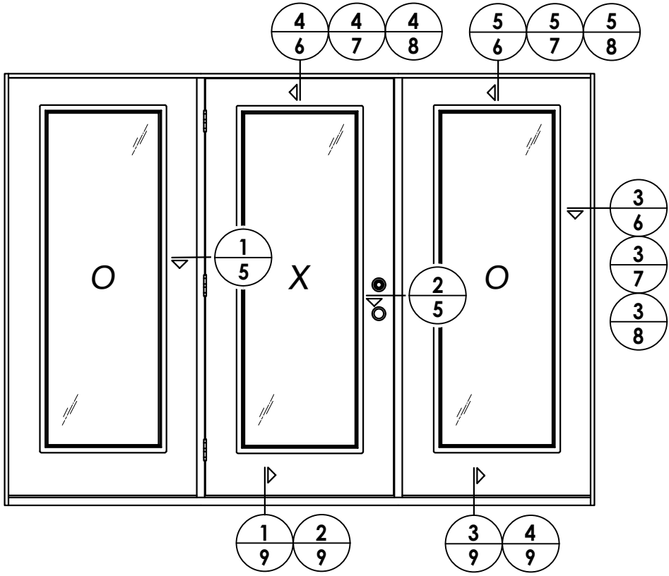
ELEVATION OXO
