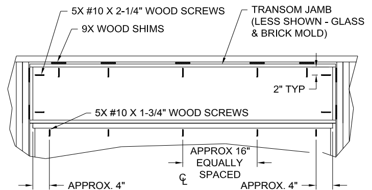
Fig. 2e (Rectangular Transom)
